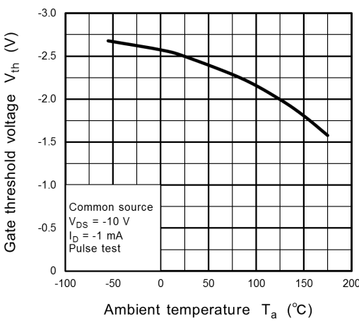
Fig. 8.9 V_{th} - T_a
