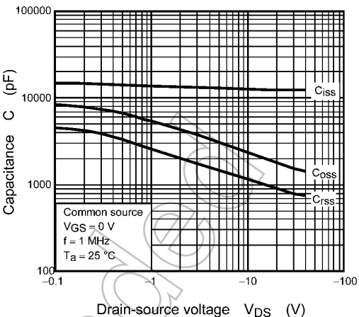
Fig. 9.8 Capacitance - V_{DS}
