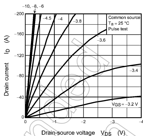
Fig. 9.2 I_D - V_{DS}
