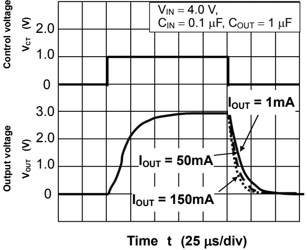
V_{OUT}=3.0V
