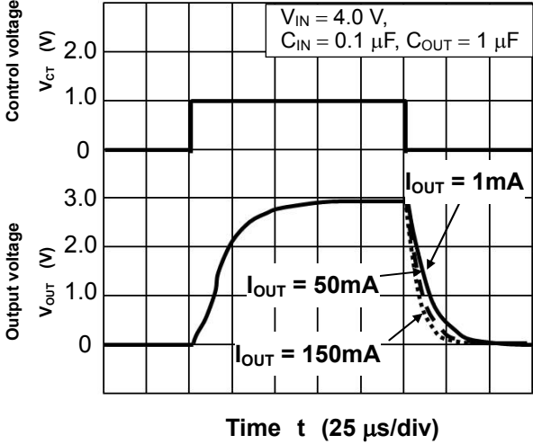
V_{OUT}=3.0V
