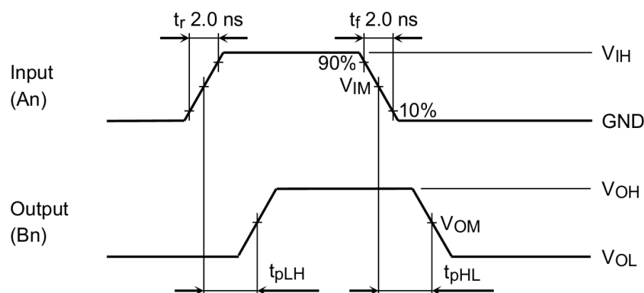
Fig. 13.1 t_{PLH} , t_{PHL}
