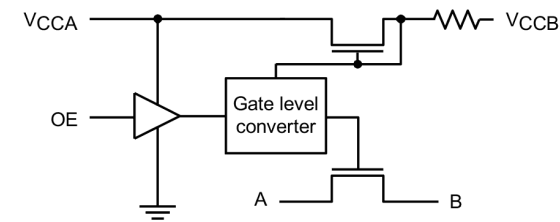
TC7SPB9306TU
