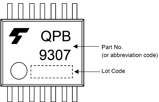
Fig. 6.4 TSSOP14
