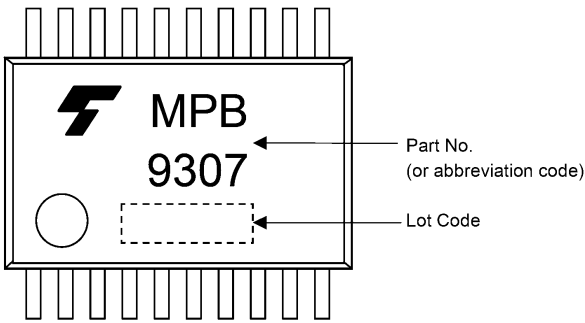
Fig. 6.2 TSSOP20
