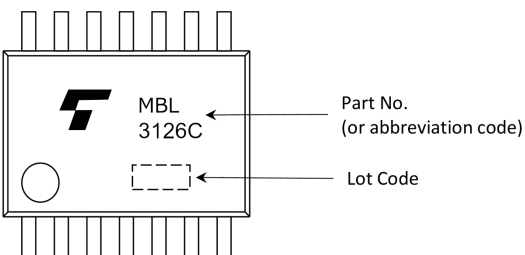
Fig. 6.4 TSSOP14
