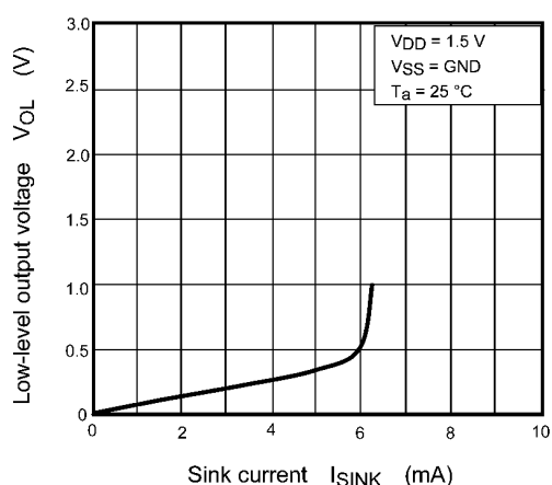
Fig. 9.1 V_{OL} - I_{SINK}
