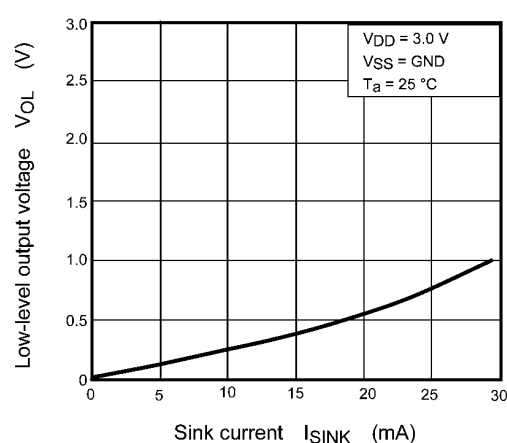
Fig. 9.2 V_{OL} - I_{SINK}
