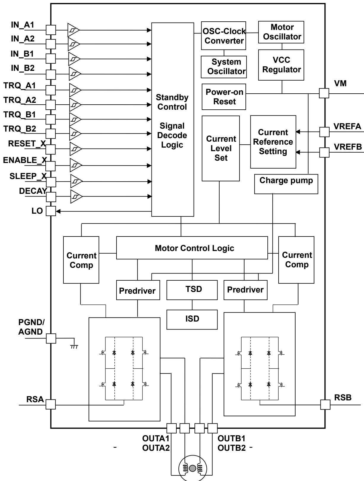
図 4 Block diagram
