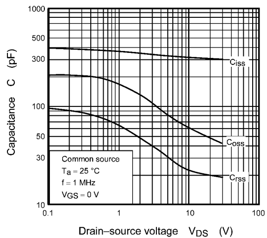
Fig. 7.10 C - V_{DS}
