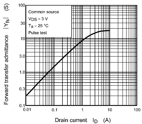
Fig. 7.8 |Y_{fs}| - I_D
