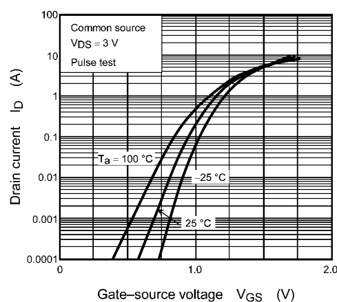
Fig. 7.2 I_D - V_{GS}
