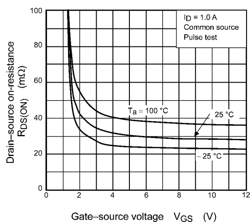
Fig. 7.3 R_{DS(ON)} - V_{GS}
