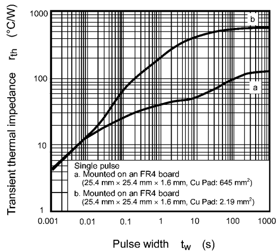
Fig. 7.13 r_{th} - t_w
