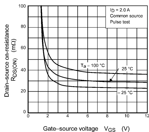
Fig. 7.4 R_{DS(ON)} - V_{GS}
