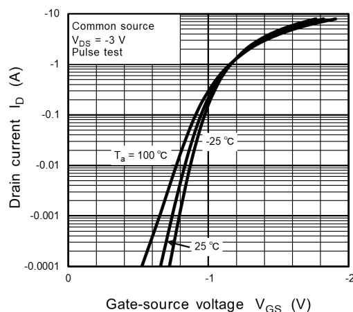
Fig. 8.2.2 I_D - V_{GS}
