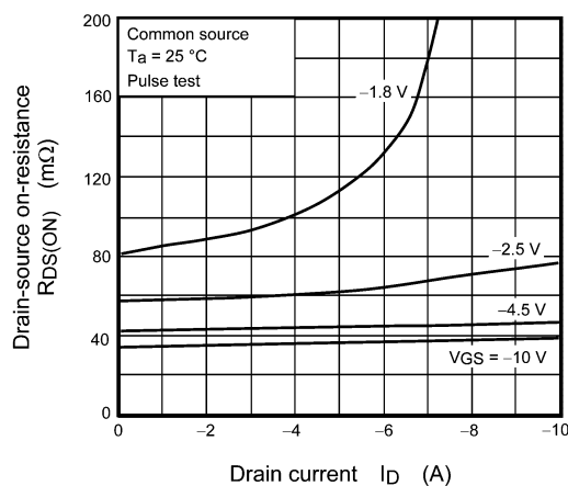
Fig. 8.2.4 R_{DS(ON)} - I_D
