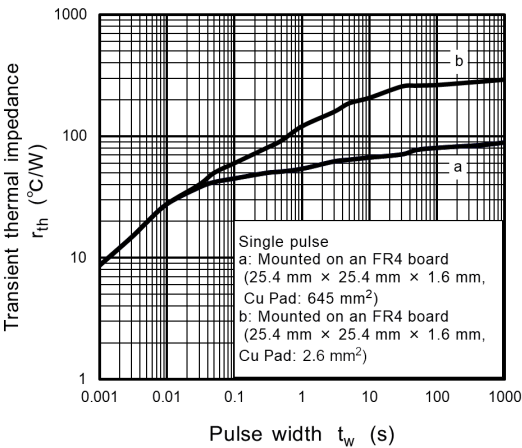
Fig. 8.3.1 r_{th} - t_w
