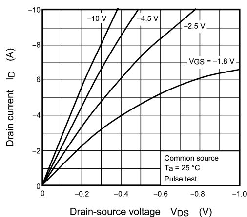
Fig. 8.2.1 I_D - V_{DS}
