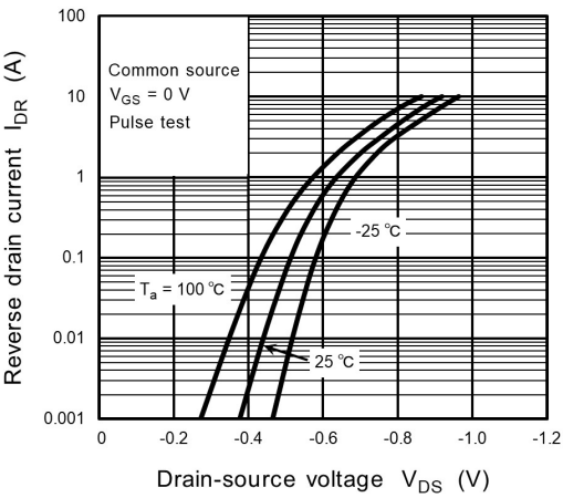
Fig. 8.1.8 I_{DR} - V_{DS}
