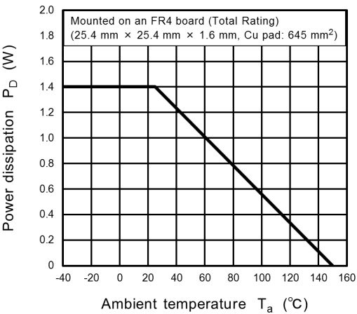
Fig. 8.3.2 P_D - T_a
