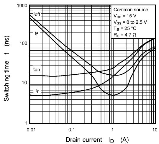
Fig. 8.1.10 t - I_D
