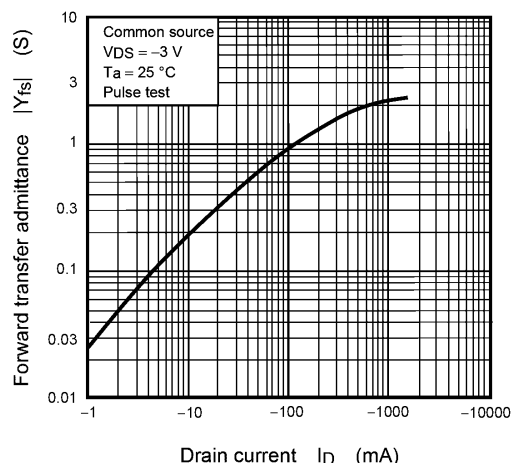
Fig. 7.2.8 |Y_{fs}| - I_D
