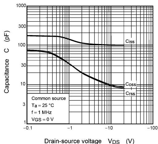
Fig. 7.2.10 C - V_{DS}
