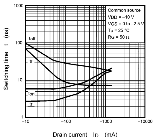
Fig. 7.2.11 t - I_D
