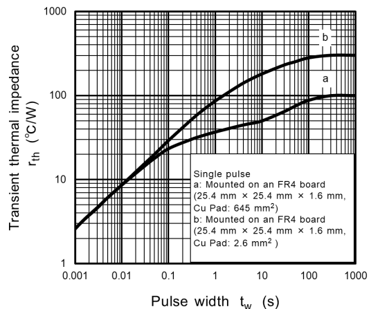
Fig. 8.12 r_{th} - t_w
