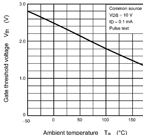
Fig. 8.6 V_{th} - T_a
