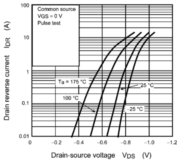
Fig. 8.7 I_{DR} - V_{DS}
