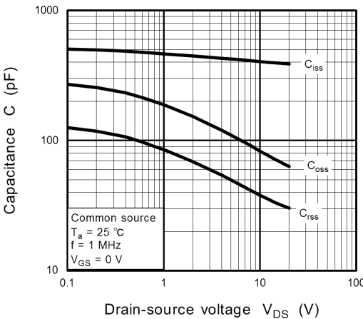
Fig. 8.8 C - V_{DS}
