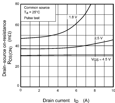
Fig. 8.5 R_{DS(ON)} - I_D
