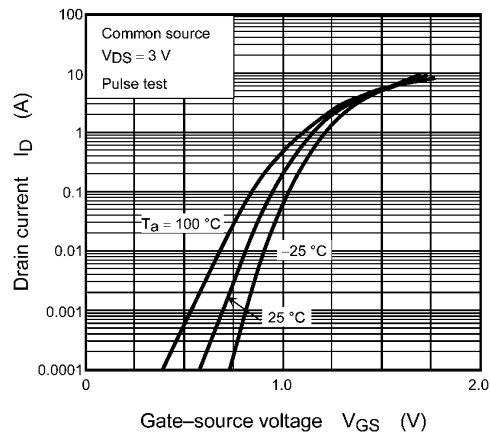
Fig. 8.2 I_D - V_{GS}
