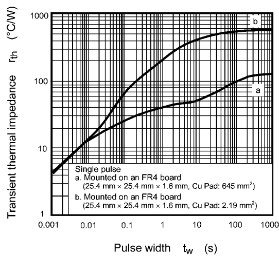
Fig. 8.13 r_{th} - t_w
