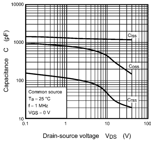
Fig. 8.9 C - V_{DS}
