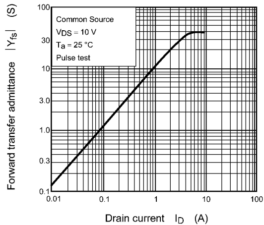
Fig. 8.8 |Y_{fs}| - I_D
