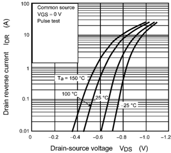
Fig. 8.7 I_{DR} - V_{DS}
