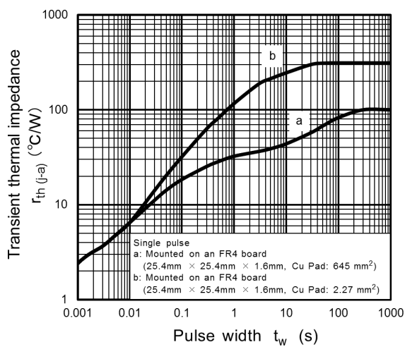
Fig. 8.11 r_{th} - t_w
