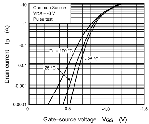
Fig. 8.2 I_D - V_{GS}
