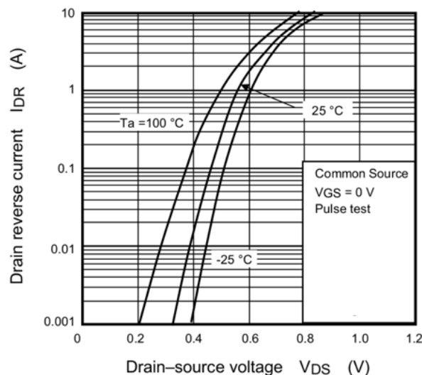
Fig. 8.8 I_{DR} - V_{DS}
