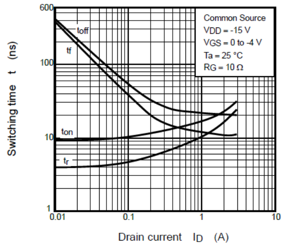
Fig. 7.10 t - I_D
