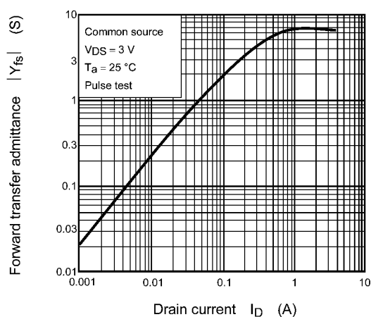
Fig. 7.1.8 |Y_{fs}| - I_D
