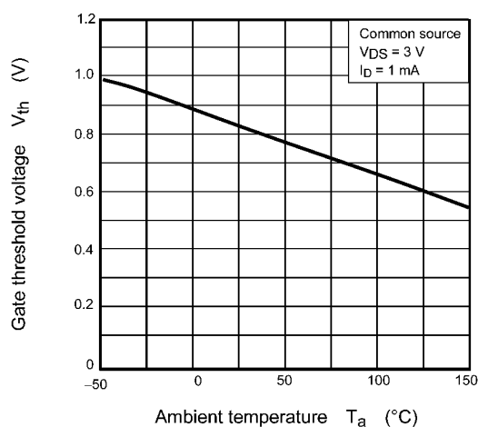
Fig. 7.1.7 V_{th} - T_a
