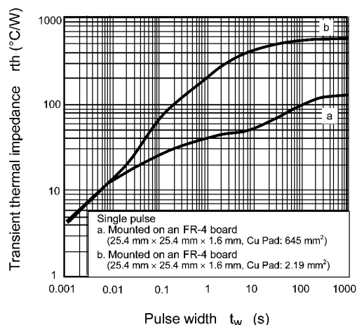
Fig. 7.3.1 r_{th} - t_w
