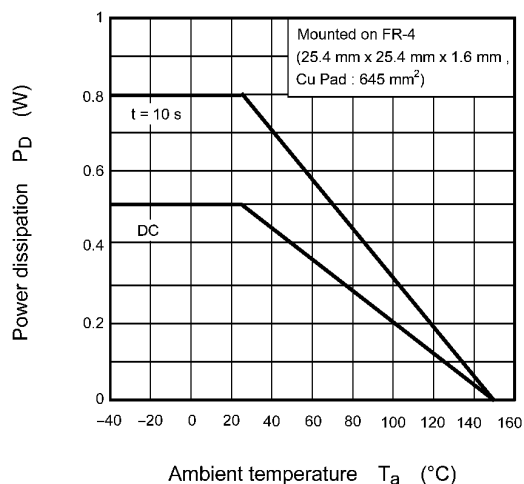
Fig. 7.1.12 P_D - T_a
