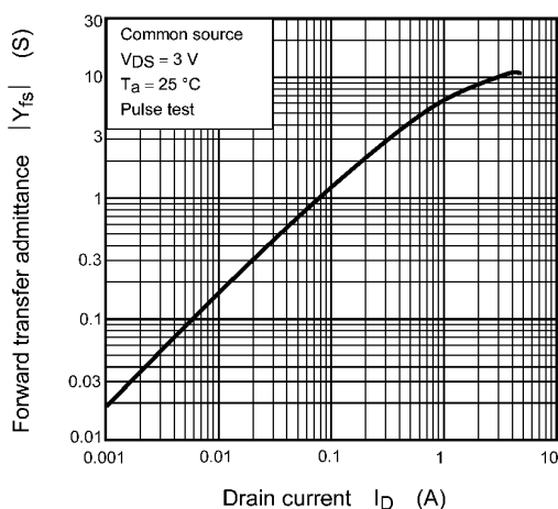
Fig. 7.1.7 |Y_{fs}| - I_D
