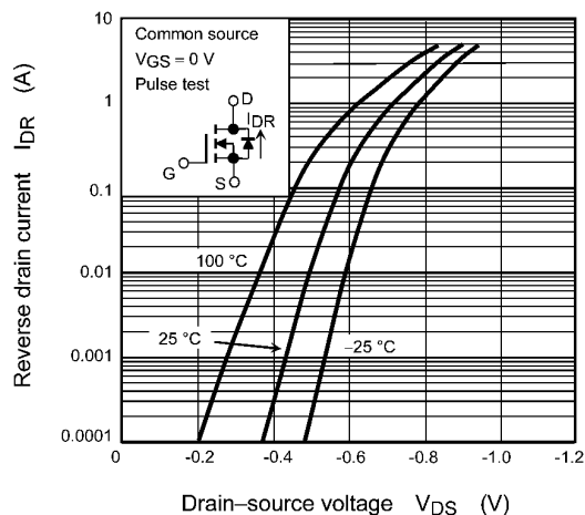
Fig. 7.1.8 I_{DR} - V_{DS}
