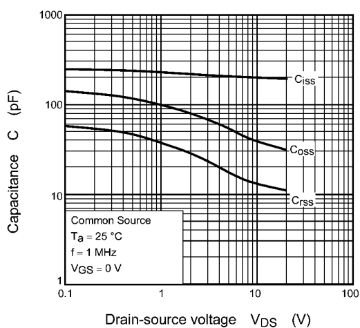
Fig. 7.1.9 C - V_{DS}
