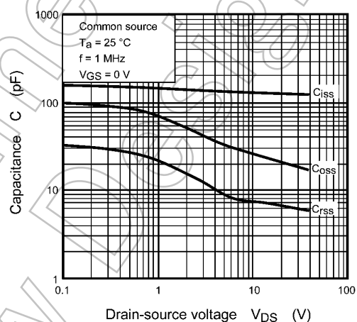
Fig. 7.10 C - V_{DS}
