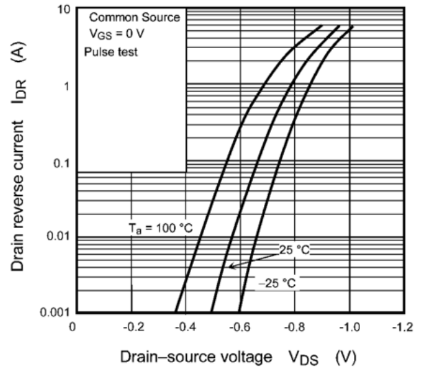
Fig. 7.8 I_{DR} - V_{DS}
