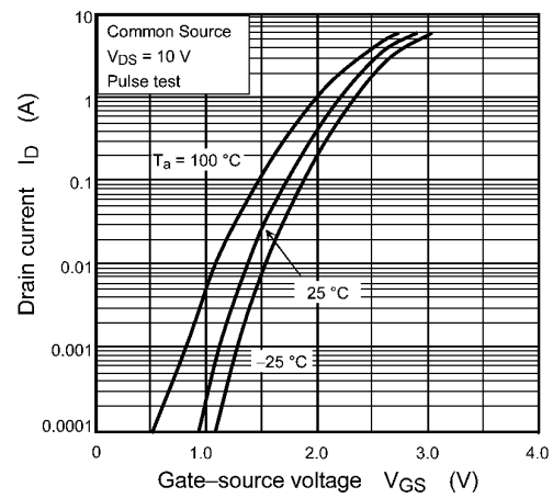
Fig. 7.2 I_D - V_{GS}
