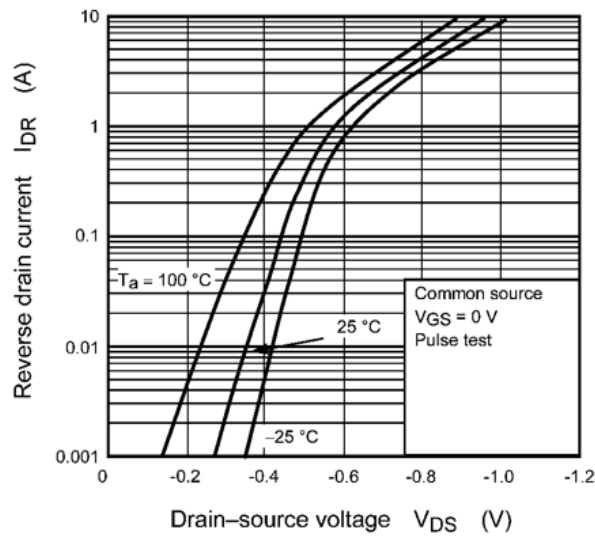
Fig. 7.9 I_{DR} - V_{DS}
