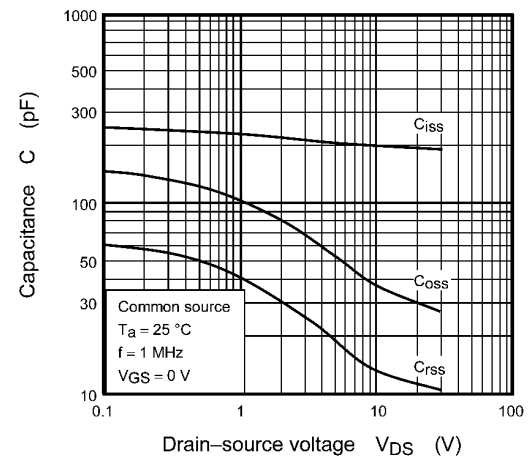
Fig. 7.10 C - V_{DS}
