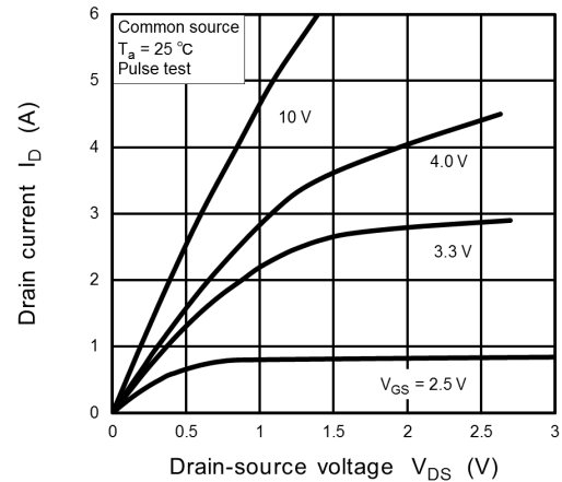
Fig. 7.2 I_D - V_{DS}
