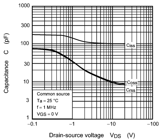
Fig. 8.10 C - V_{DS}
