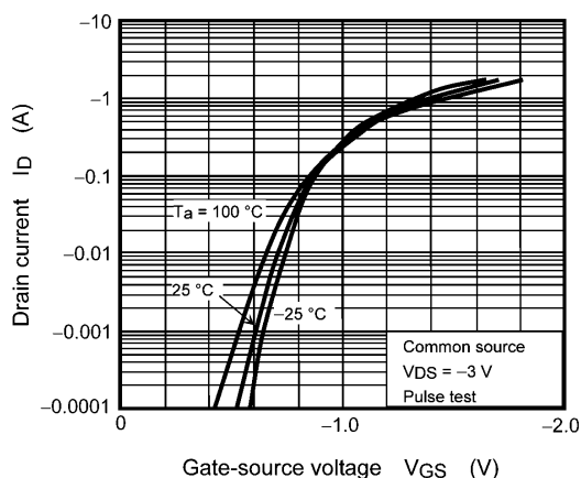
Fig. 8.2 I_D - V_{GS}
