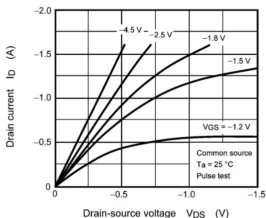
Fig. 8.1 I_D - V_{DS}
