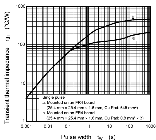
Fig. 8.12 r_{th} - t_w
