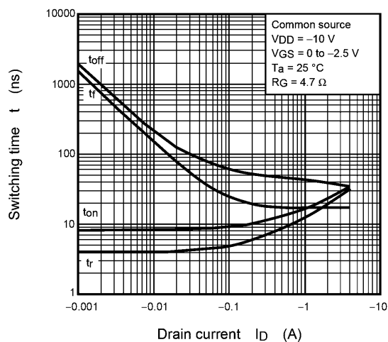
Fig. 8.10 t - I_D
