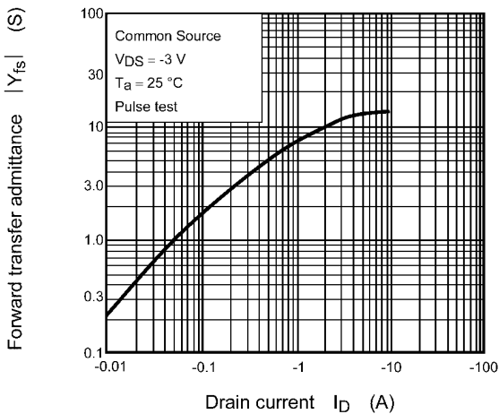
Fig. 8.8 |Y_{fs}| - I_D
