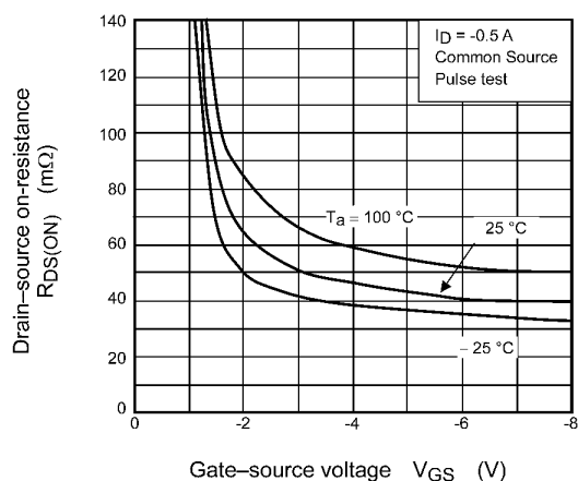
Fig. 8.3 R_{DS(ON)} - V_{GS}
