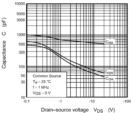
Fig. 8.10 C - V_{DS}
