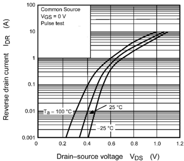
Fig. 8.9 I_{DR} - V_{DS}
