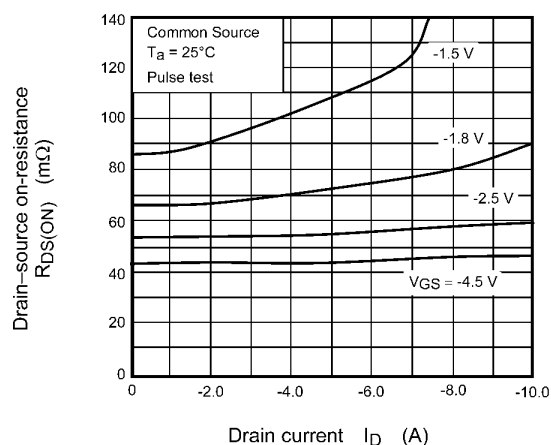
Fig. 8.5 R_{DS(ON)} - I_D
