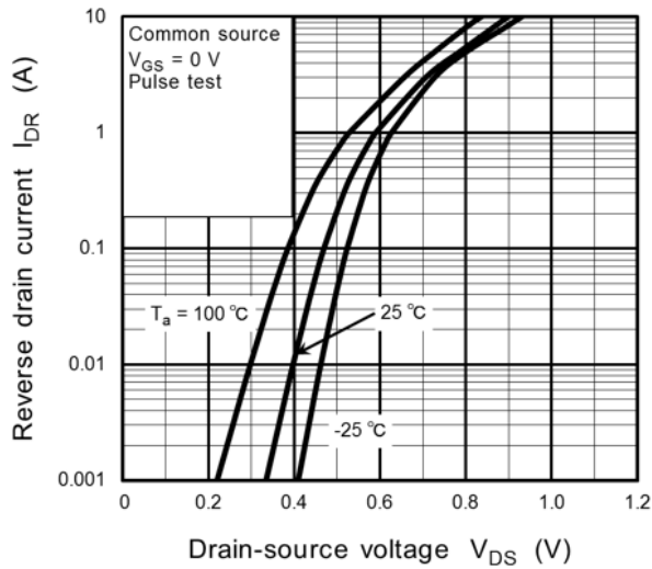
Fig. 7.7 I_{DR} - V_{DS}
