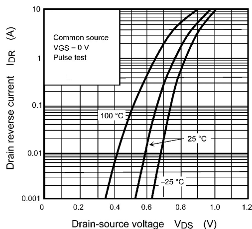
Fig. 9.7 I_{DR} - V_{DS}
