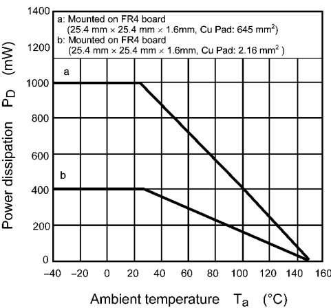
Fig. 9.13 P_D - T_a
