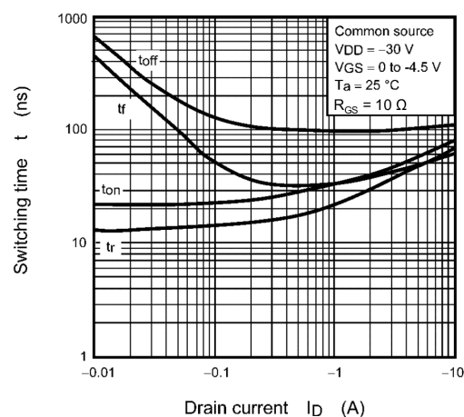
Fig. 9.10 t - I_D
