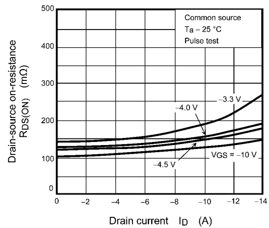
Fig. 9.4 R_{DS(ON)} - I_D
