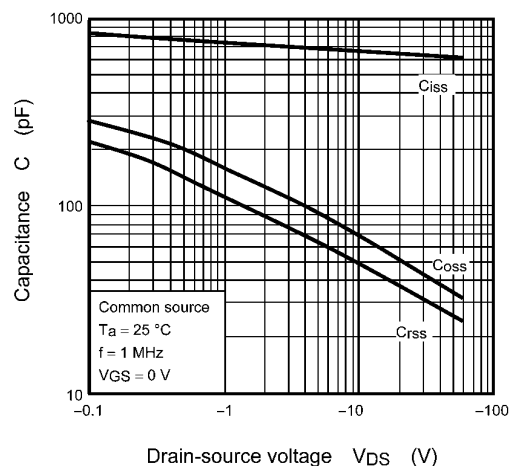
Fig. 9.8 C - V_{DS}
