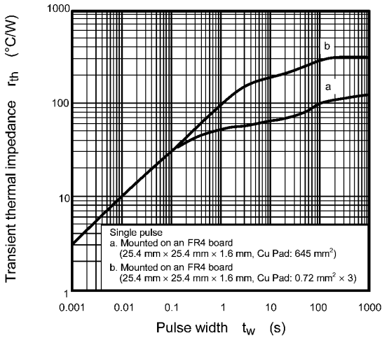
Fig. 7.13 r_{th} - t_w
