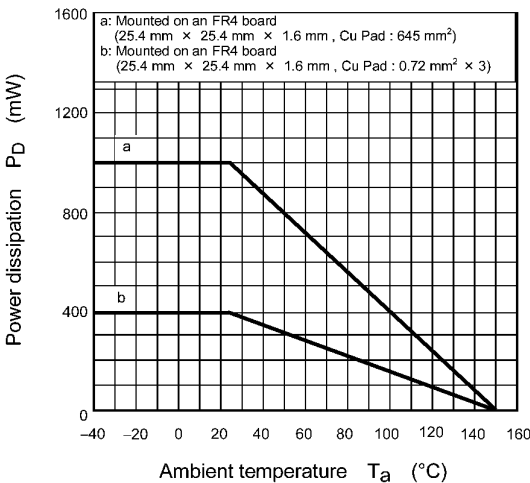
Fig. 7.14 P_D - T_a
