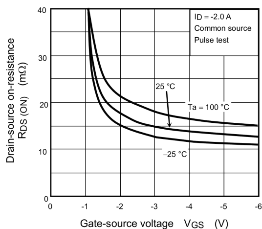
Fig. 7.4 R_{DS(ON)} - V_{GS}
