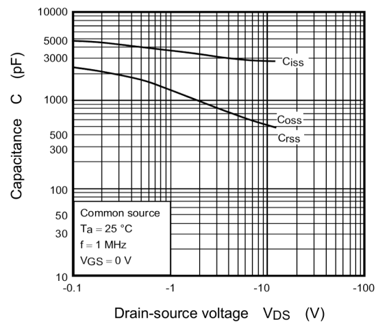
Fig. 7.10 C - V_{DS}
