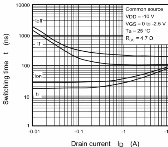
Fig. 7.11 t - I_D
