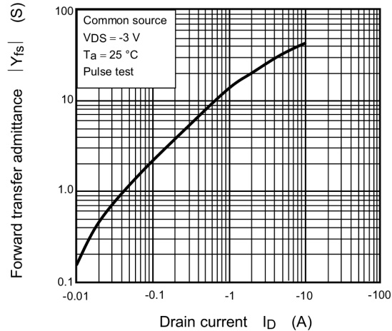
Fig. 7.8 |Y_{fs}| - I_D
