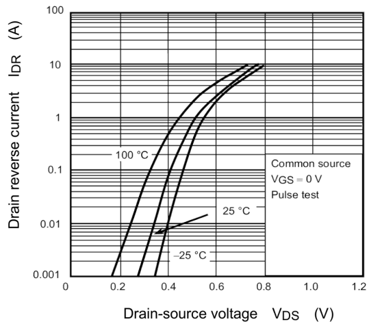
Fig. 7.9 I_{DR} - V_{DS}
