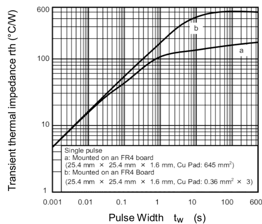
Fig. 7.13 r_{th} - t_w
