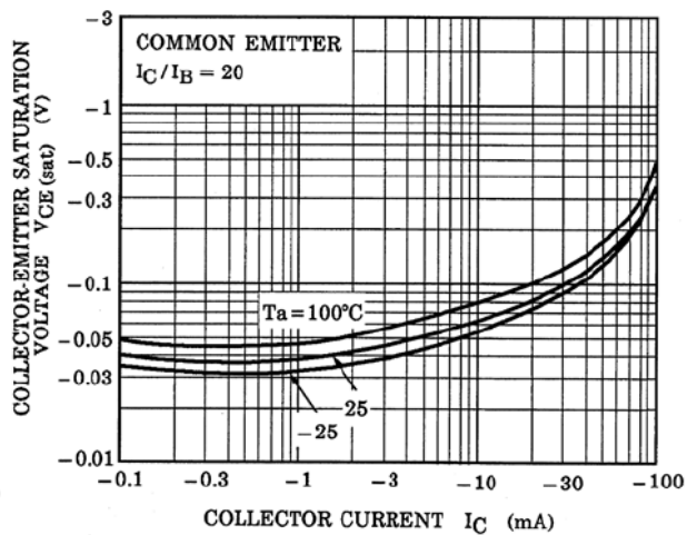
Fig. 13.8 Q2 V_{CE(sat)}-I_C
