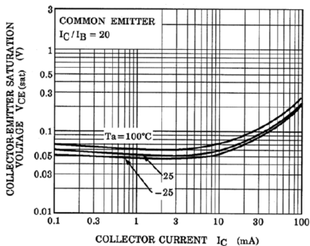
Fig. 13.7 Q1 V_{CE(sat)}-I_C
