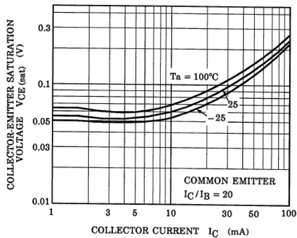
Fig. 13.7 Q1 V_{CE(sat)}-I_C
