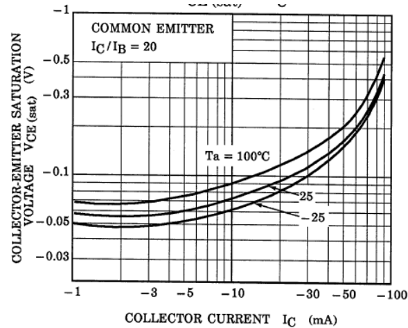
Fig. 13.8 Q2 V_{CE(sat)}-I_C
