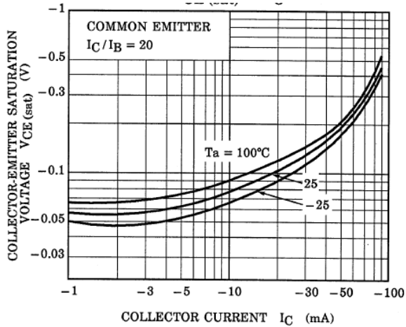
Fig. 13.8 Q2 V_{CE(sat)}-I_C
