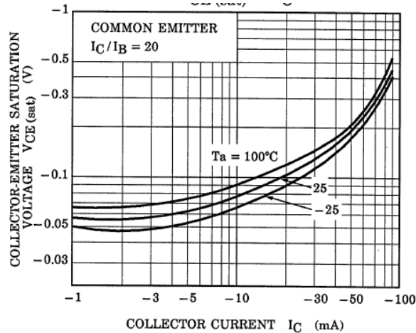
Fig. 13.8 Q2 V_{CE(sat)}-I_C
