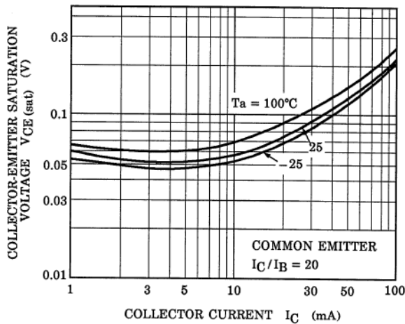
Fig. 13.7 Q1 V_{CE(sat)}-I_C
