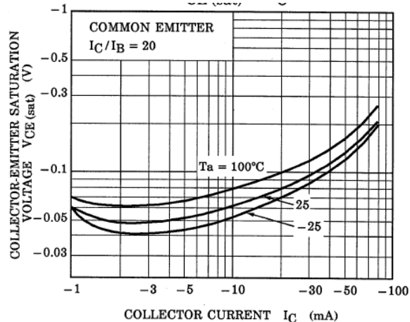
Fig. 13.8 Q2 V_{CE(sat)}-I_C
