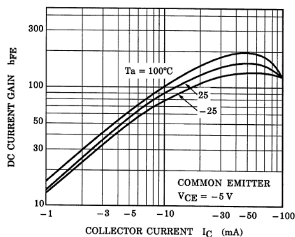
Fig. 14.6 Q2 h_{FE} - I_C
