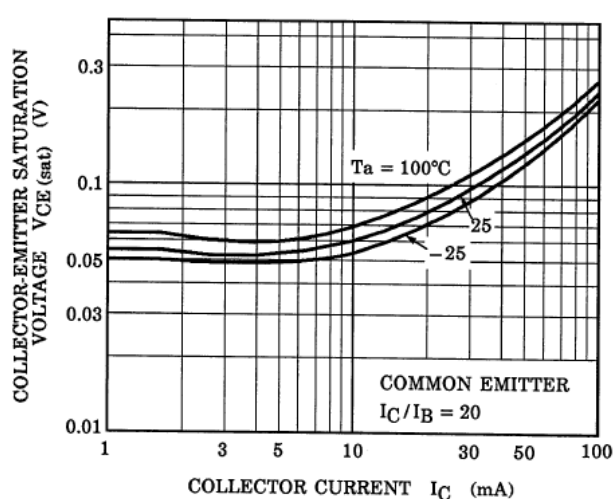
Fig. 13.8 Q2 V_{CE(sat)}-I_C
