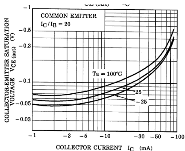
Fig. 13.7 Q1 V_{CE(sat)}-I_C
