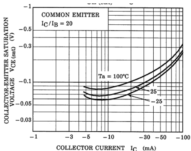
Fig. 10.19 RN2901FE V_{CE(sat)}-I_C
