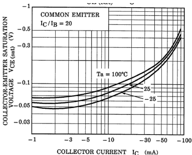
Fig. 10.23 RN2905FE V_{CE(sat)}-I_C
