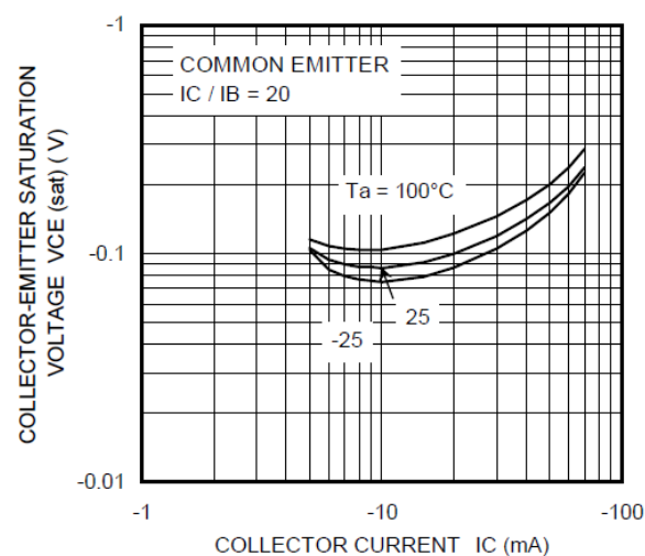
Fig. 10.19 RN2417 V_{CE(sat)}-I_C
