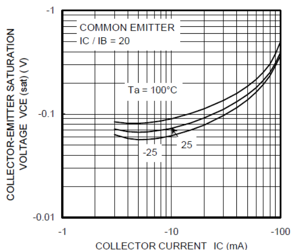
Fig. 10.17 RN2415 V_{CE(sat)}-I_C
