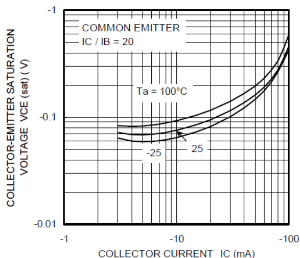
Fig. 10.16 RN2414 V_{CE(sat)}-I_C
