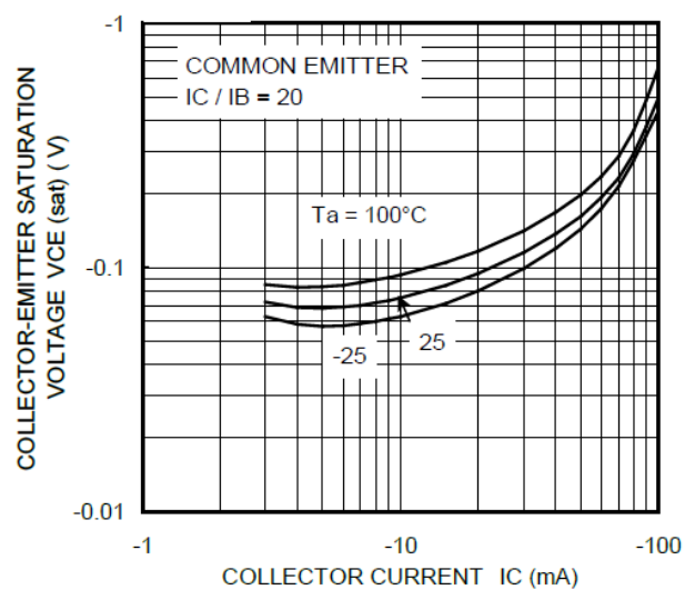
Fig. 10.18 RN2316 V_{CE(sat)}-I_C
