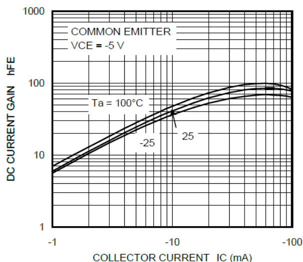
Fig. 10.14 RN2317 h_{FE}-I_C
