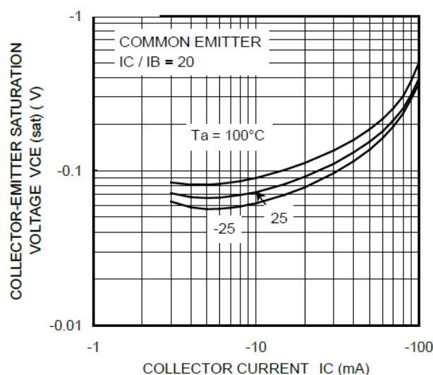
Fig. 10.17 RN2315 V_{CE(sat)}-I_C
