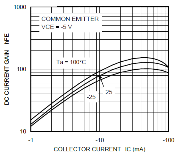
Fig. 10.13 RN2316 h_{FE}-I_C
