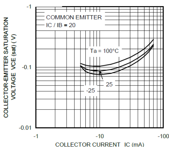
Fig. 10.19 RN2117 V_{CE(sat)}-I_C
