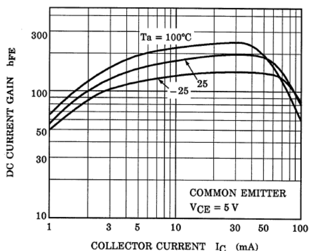
Fig. 10.17 RN1905 h_{FE}-I_C
